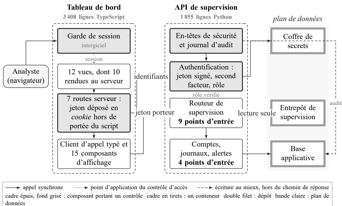
FIG. 21. Architecture interne des deux logiciels écrits : composants, frontières de déploiement et points d'application du contrôle d'accès. Le rôle est vérifié sur les treize points d'entrée de données de l'API — neuf de supervision et quatre de gestion — et jamais dans le tableau de bord, qui ne détient aucune autorisation propre ; l'échec de l'écriture d'audit est absorbé et ne fait jamais échouer la requête de l'analyste.
