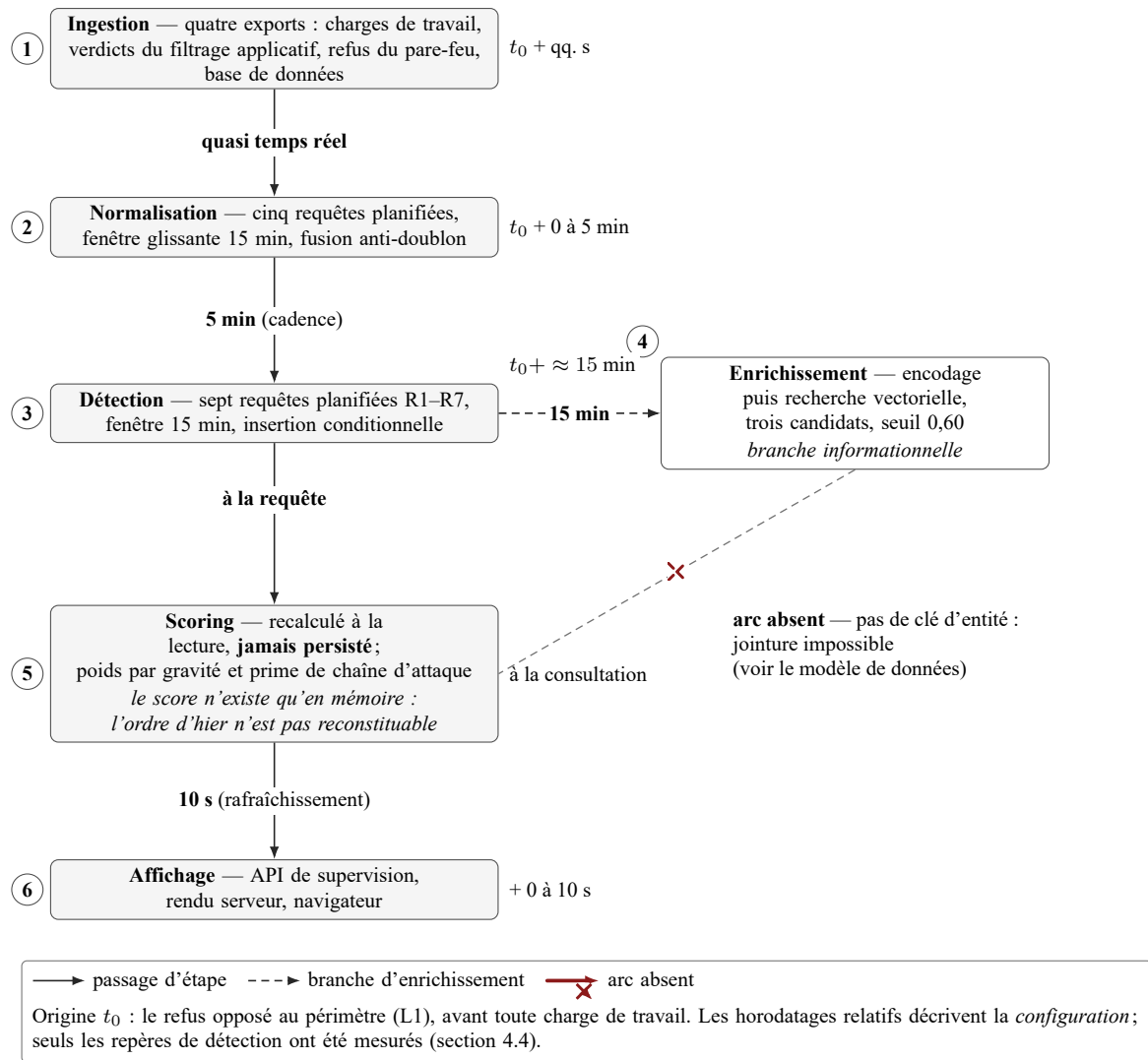
FIG. 13. Cycle de vie de la donnée de sécurité : six étapes, le budget de latence porté par les cadences et l'horodatage relatif de chaque étape. Le délai entre l'événement et son affichage est fait d' attentes d'ordonnanceur et non de temps de traitement : trois attentes s'additionnent (5 + 5 + 15 min), et aucune puissance de calcul ne les réduirait. La branche d'enrichissement n'alimente pas le calcul de score — impasse fonctionnelle assumée.
