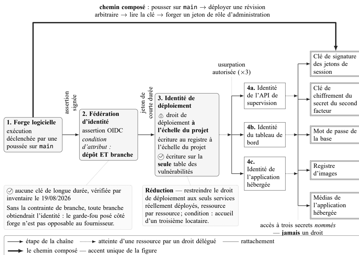
FIG. 17. Chaînes de délégation d'identité : ce qu'un droit de déploiement à l'échelle du projet rend atteignable. Aucun droit pris isolément n'est anormal — la fédération est durcie par une condition d'attribut portant sur le dépôt et sur la branche, sans clé de longue durée, et l'écriture à l'entrepôt est bornée à une seule table. Le risque naît de la composition : c'est la portée du droit de déploiement, en aval, qui porte le risque résiduel, non la fédération, en amont.
