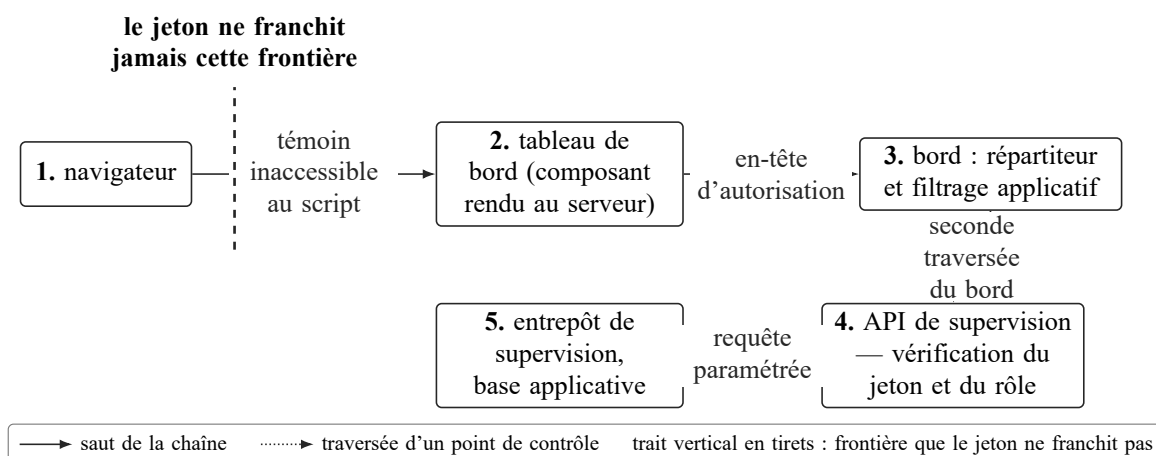
FIG. 22. Chaîne de données d'une vue du tableau de bord : les cinq sauts, et la frontière que le jeton ne franchit pas. L'autorité d'autorisation est l'API de supervision, qui vérifie le jeton et le rôle ; l'identité du tableau de bord ne détient aucune autorisation sur les données.
