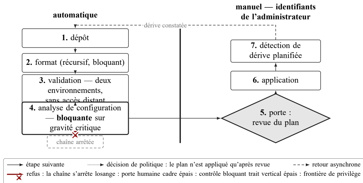
FIG. 20. Chaîne de provisionnement de l'infrastructure : la frontière automatique/manuel est un choix de privilège , non un degré d'achèvement — la partie automatisée n'a, par construction, aucun accès au fournisseur cloud.
