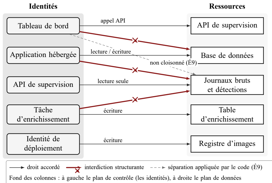
FIG. 16. Plan d'identité : droits accordés et interdictions structurantes (cinq identités). Ni l'application hébergée ni la tâche d'enrichissement ne peuvent écrire sur les preuves (scénario SO16, test T11); le tableau de bord passe par l'API de supervision, mais son identité conserve un droit de lecture sur l'entrepôt — c'est l'écart É9.
