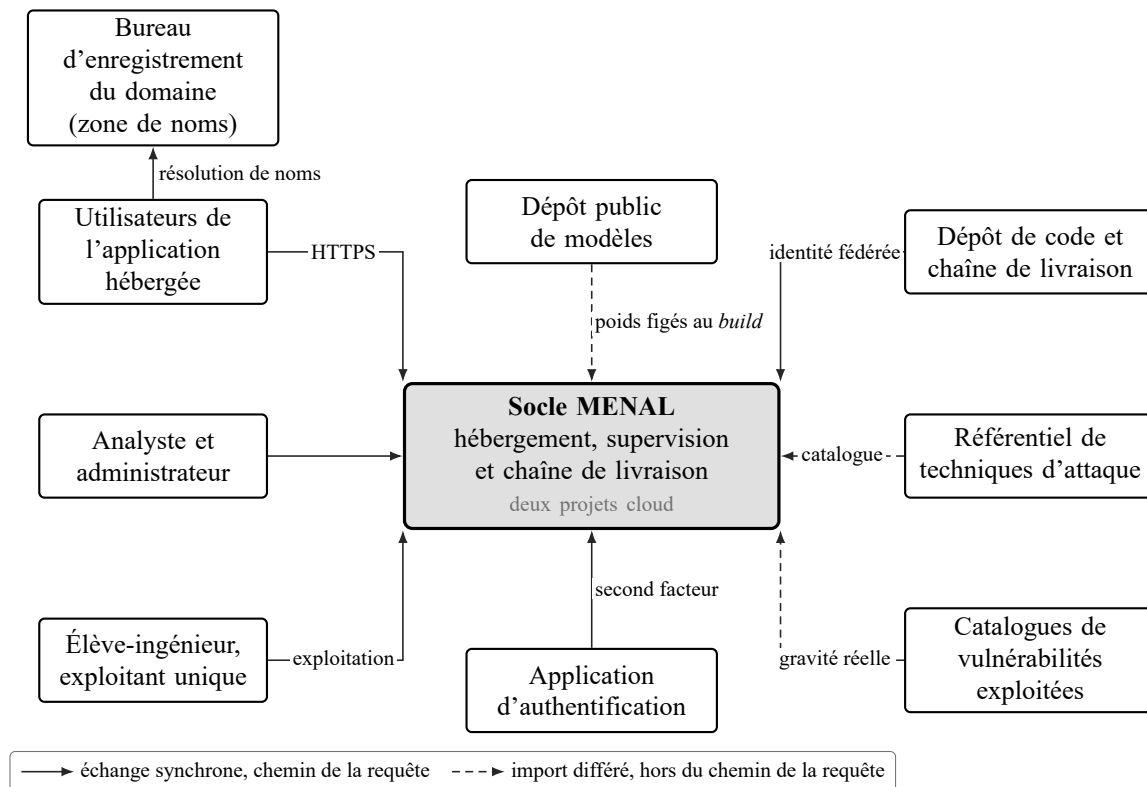
FIG. 8. Vue de contexte : le socle, ses acteurs et les six systèmes extérieurs dont il dépend — trois imports différés portent le risque de chaîne d’approvisionnement, la zone de noms échappe seule à la description en code (É10)
