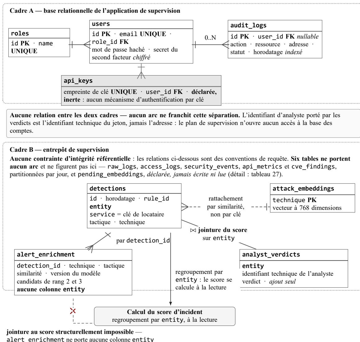
FIG. 14. Modèle de données des deux systèmes de stockage : ce que les clés permettent, et la jointure que leur absence interdit. L'impossibilité de corréler le rattachement sémantique au score d'incident est une propriété du schéma et non un choix d'algorithme — une colonne manquante suffit à l'expliquer — et les deux systèmes de stockage sont volontairement disjoints.
