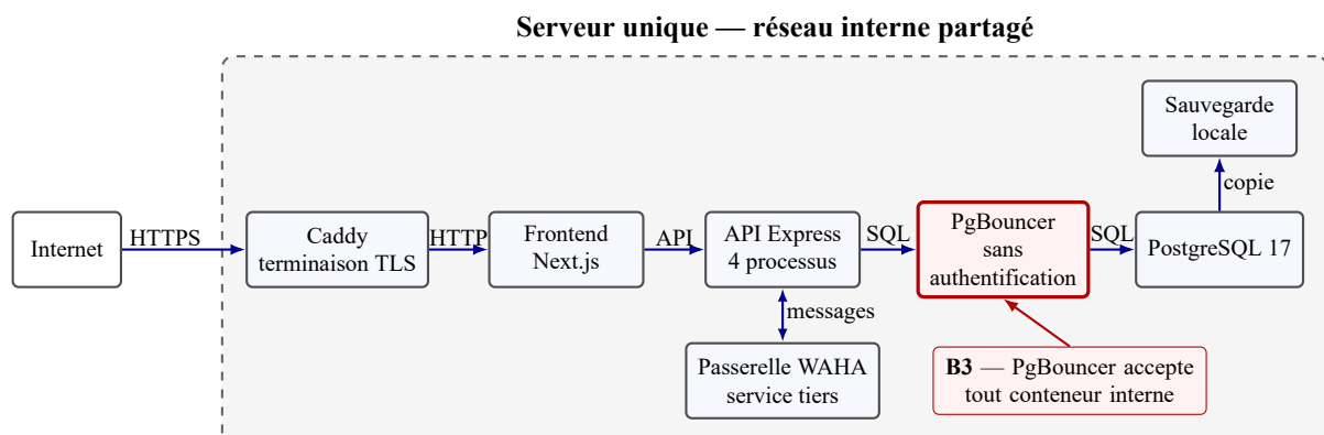
FIG. 4. Modèle de sécurité avant le projet : périmètre unique en entrée, confiance implicite à l'intérieur. Tout composant présent sur le réseau interne est traité comme légitime — c'est la carence C1.
