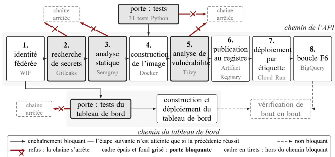
FIG. 19. Chaîne de livraison applicative. Chemin de l'API : huit étapes, dont trois portes bloquantes, plus la porte de tests qui conditionne la construction ; chemin du tableau de bord : sa propre porte. La vérification de bout en bout suit le déploiement et ne le défait pas — c'est une vérification, non une porte. Les cas de refus sont décrits en section 5.2.6 ; deux d'entre eux portent un protocole numéroté, T8 et T10, dont le chapitre 6 donne le verdict daté.
