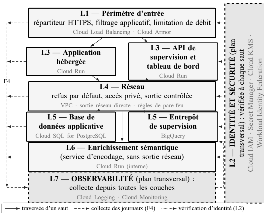
FIG. 9. Modèle en couches : cinq couches empilées (L1, L3, L4, L5, L6) et deux plans transversaux (L2, L7), dont la bordure en tirets marque la portée. La résolution de noms ne figure pas en L1 : elle est une dépendance externe (figure 8).
