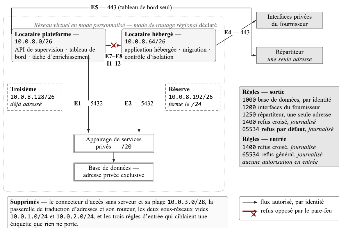
FIG. 12. Topologie réseau après la refonte appliquée du 11 au 25/08/2026 — le réseau en service à 25/08/2026, à comparer à la figure 11. Les charges de travail émettent depuis un sous-réseau : le pare-feu leur est applicable, et aucune autorisation ne comporte de plage source.
