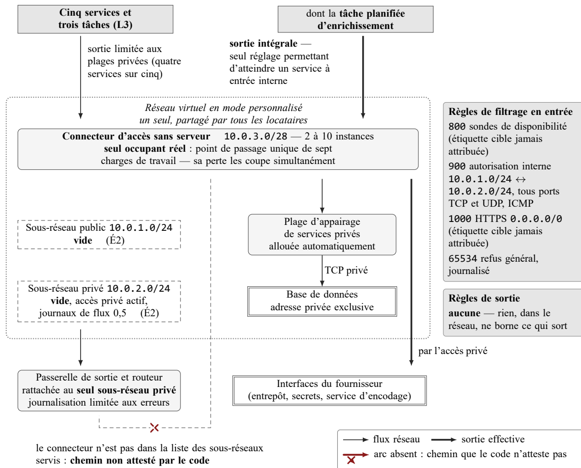
FIG. 11. Topologie réseau avant la refonte — état du dépôt jusqu'au 11/08/2026. La sortie des charges de travail n'y était pas gouvernée par le réseau mais par le paramètre de la plateforme d'exécution : la passerelle ne desservait que le sous-réseau privé, lequel était vide, et la plage qui portait la totalité de la sortie ne lui était pas rattachée. Aucune règle de sortie n'existait : c'est le diagnostic qui a motivé D15.
